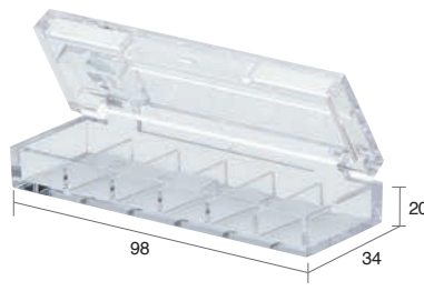
pan size : 27 x 14 C-0385
